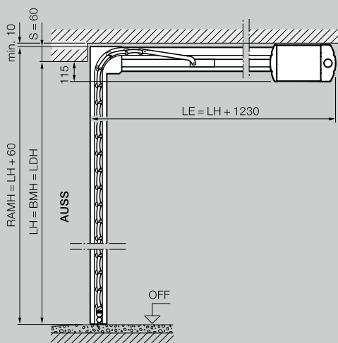
Rozsah velikostí vrat zajiždějí pod strop RollMatic OD*
